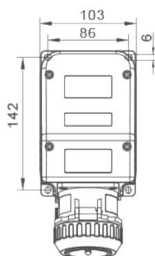
Tomada sobrepor
