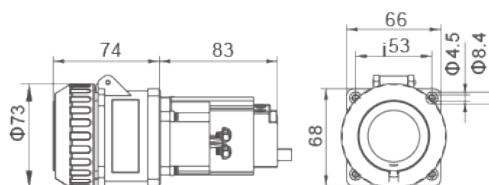
Tomada embutir
