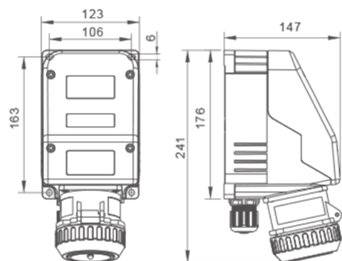
Tomada sobrepor
