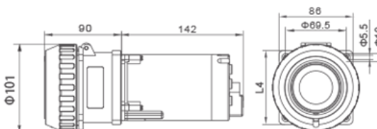
Tomada embutir
