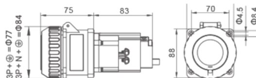
Tomada embutir
