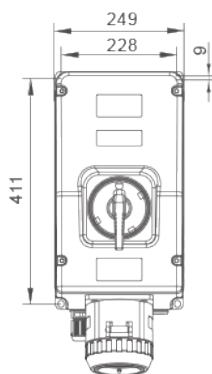
Tomada sobrepor
