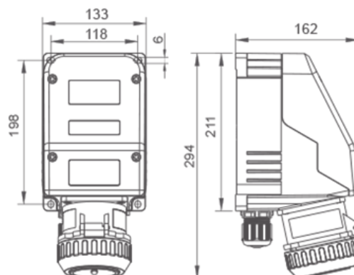
Tomada sobrepor
